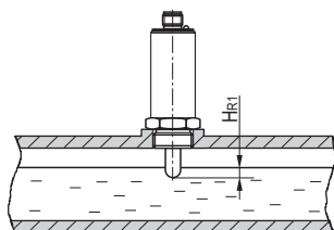
Схемы монтажа
